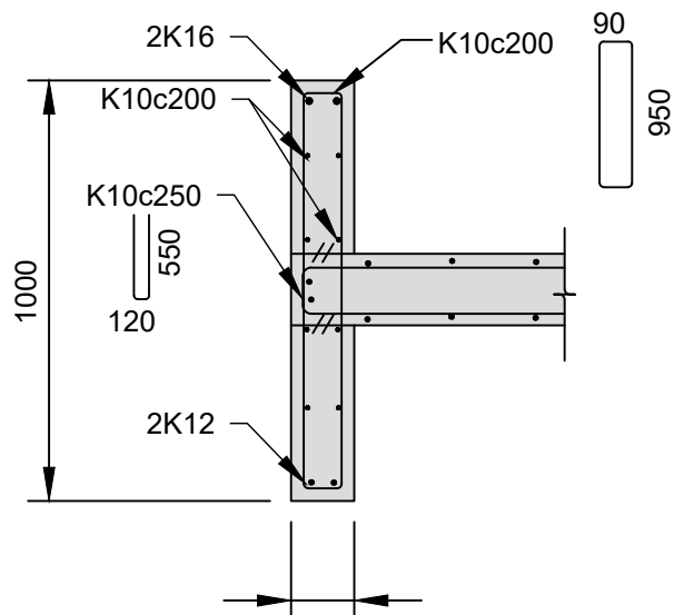
11 SNÍÐ 002 1:20 11* SAMBÆRILEGT 11** YFIR HORN GLUGGA, ÚTKRAGANDI
